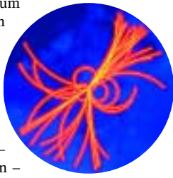
Teilchenpuren: Computersimulation des Zerfalls eines Higgs-Teilchens im Detektor
